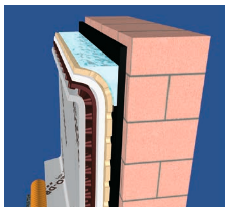
Accumulo d'acqua di ruscellamento lungo la facciata.
