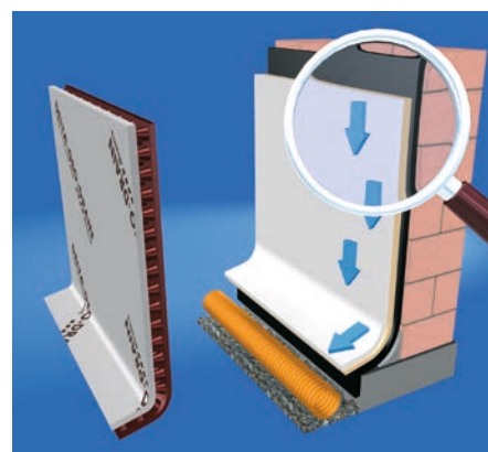
L'acqua è in seguito drenata grazie ad un geotessile filtrante (strato 2).
