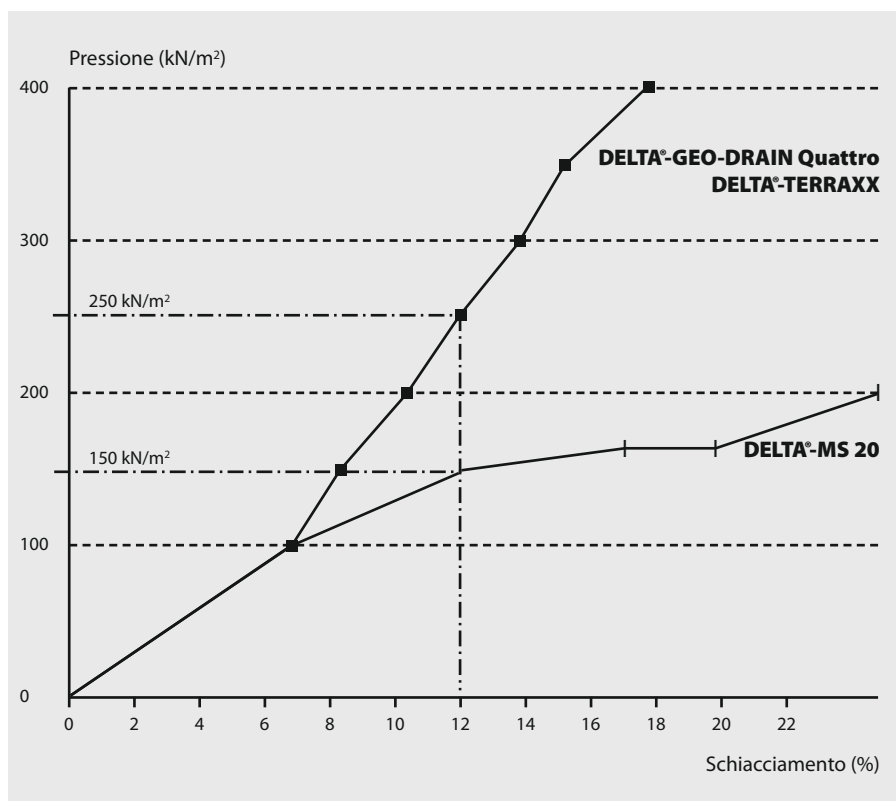
Schiacciamento percentuale di DELTA®-MS, DELTA®-MS 20, DELTA®-TERRAXX e DELTA®-GEO-DRAIN Quattro con carichi di breve durata.
