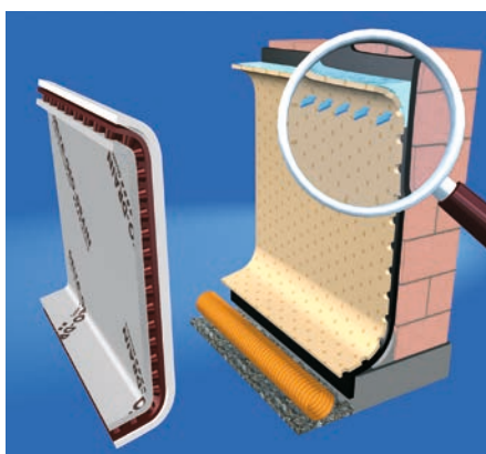
L'acqua presente tra DELTA®-GEO-DRAIN Quattro e l'impermeabilizzazione può attraversare lo strato liscio di scorrimento grazie a micro-fori.
