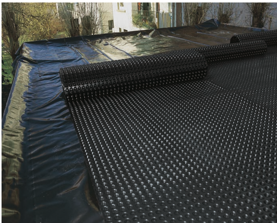
DELTA®-FLORAXX – Posa in opera ottimale.
