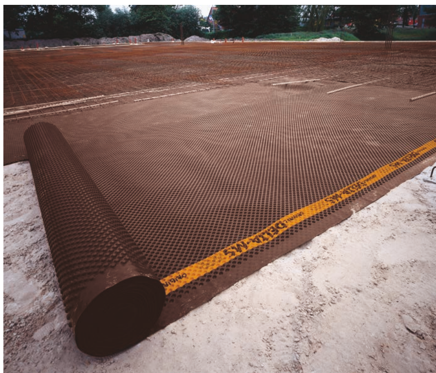
La membrana viene semplicemente srotolata sullo strato di sabbia.
