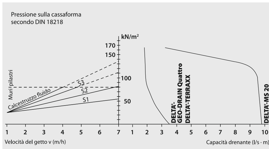
Capacità drenante delle membrane DELTA® durante la fase di getto (diagramma secondo DIN 18218). S3: cls semifluido; S2: cls plastico; S1: cls umido
