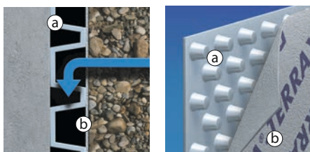
a) membrana alveolare b) geotessile integrato
