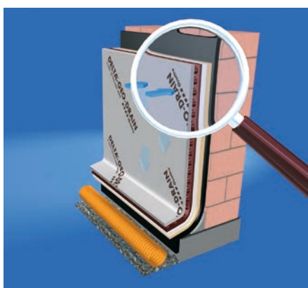
Il secondo strato geotessile permette di filtrare l'acqua proveniente dal suolo evitando l'intasamento della struttura alveolare drenate.
