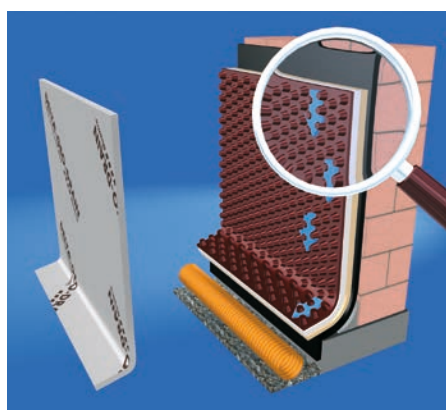
I rilievi formano una rete di canali che permettono il drenaggio verticale dell'acqua proveniente dal terreno (strato 3).
