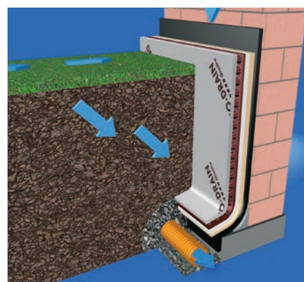
DELTA®-GEO-DRAIN Quattro: protezione a quattro strati efficace contro tutte le infiltrazioni d'acqua.
