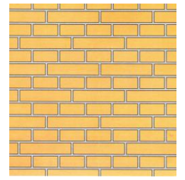
A BLOCCO / BLOCK BOND
