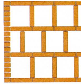
CON MATTONI DI LISTA E COLTELLO / ORTHOGONAL
