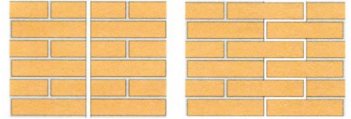
I DUE FONDAMENTALI TIPI DI GIUNTO DI DILATAZIONE VERTICALE PER LE MURATURE IN MATTONI FACCIA A VISTA SONO: RETTILINEO E DENTATO
