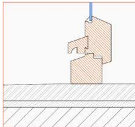
TAVOLE PER LA SIGILLATURA DEL NODO INFERIORE NELLA POSA A FILO INTERNO
