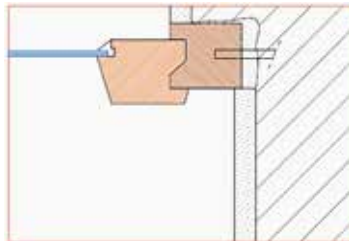
POSA CON NUOVO TELAIO CON DENTINI E FINITURA INTERNA SENZA COPRIFILO - aria 5 mm
