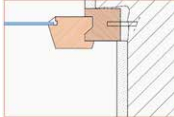
POSA IN SOVRAPPOSIZIONE SU TELAIO MURATO - aria 10 mm
