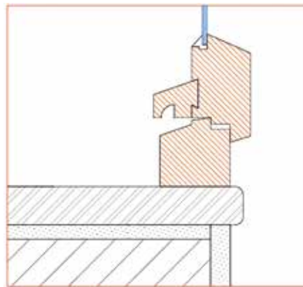
TAVOLE PER LA SIGILLATURA DEL NODO INFERIORE NELLA POSA IN MEZZERIA
