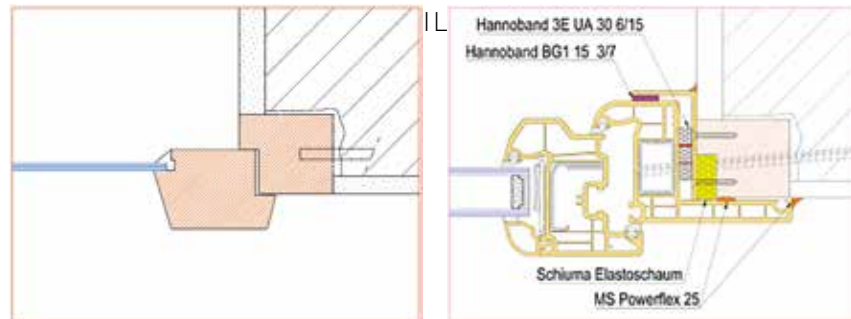
POSA IN SOVRAPPOSIZIONE SU TELAIO MURATO CON DENTINO DI BATTUTA
