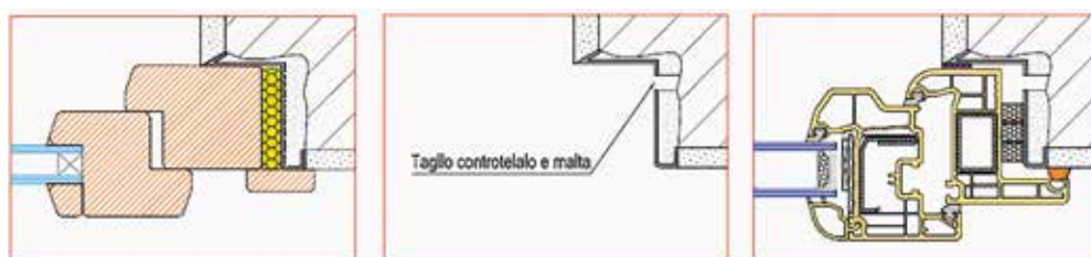
Il taglio termico del controtelaio metallico nella posa a filo muro interno : situazione di partenza, dopo il taglio e dopo la posa del serramento
