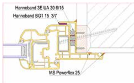
TAVOLE DI POSA DEL NUOVO TELAIO SU CONTROTELAIO "IN LUCE"
