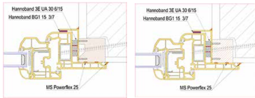
POSA IN SOVRAPPOSIZIONE SU TELAIO MURATO
