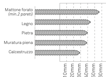
Profondità di avvitamento minima per la vite a tutto filetto su supporti di varia natura
