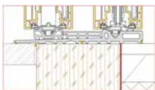
Dettaglio dei 4 cordoli di MS POWERFLEX 25 per sigillare il traverso inferiore dell'alzante scorrevole.
