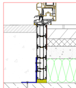
Dettaglio Nodo inferiore porta finestra.
