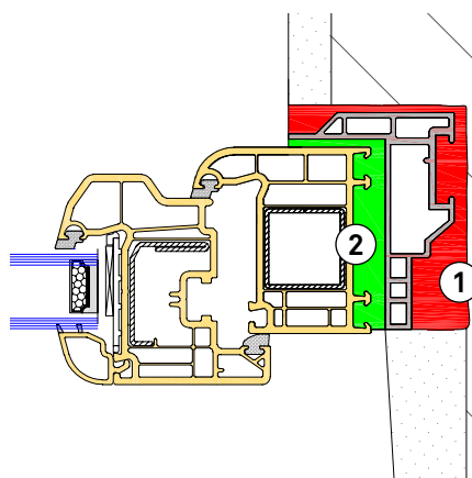
Schematizzazione del giunto primario e secondario nella posa del serramento esterno
