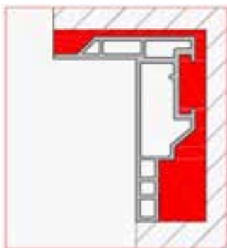
Giunto primario nodo laterale/superiore
