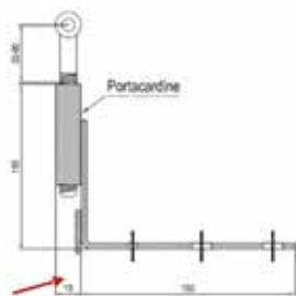
Fig. 1 disegno della staffa portacardine con le misure ed il particolare del dentino di allineamento
