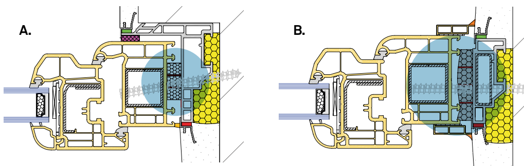
B. Posa in luce: il nastro deve soddisfare tutti i 3 piani funzionali
