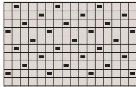
Schema E: Una tegola fermaneve ogni quinta tegola in ogni fila
